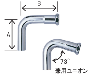
ユニオン付ベンド管
