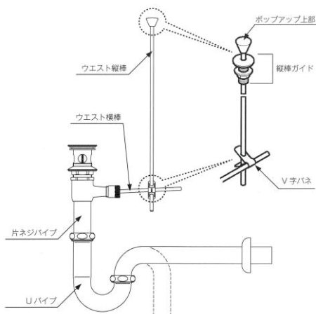
ポップアップ付Sトラップ・Pトラップ用 T7P
