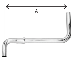
組ベンド管(ロータンク洗浄管)
