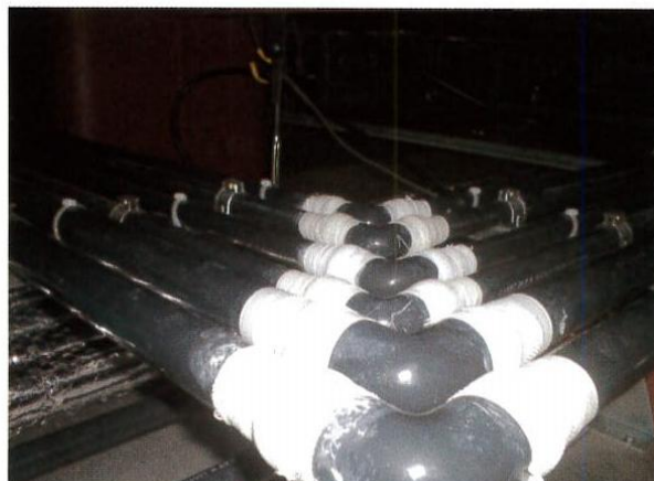
④ブチルロールの上からマホータイを巻く。
